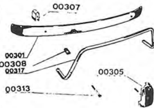
Stosstange vorne
